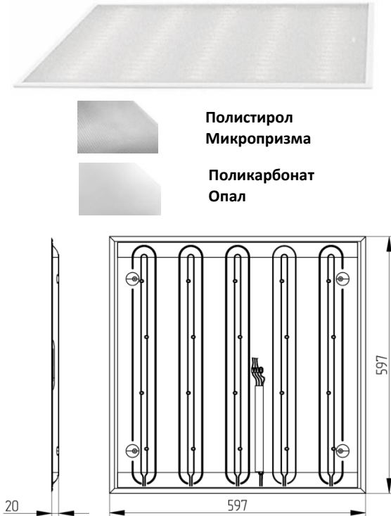
Рисунок 1 – Внешний вид и габаритные размеры.
