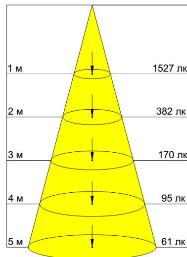
Опал 120°
