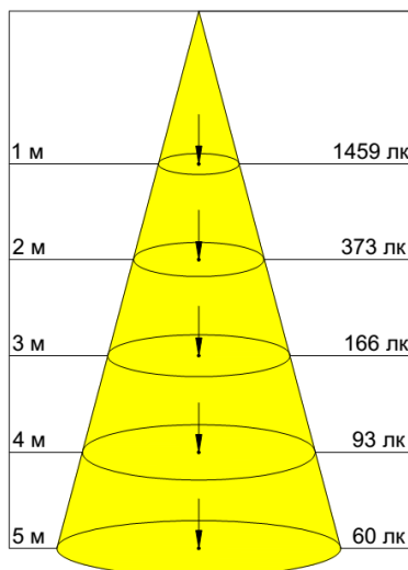
Микропризма 120°
