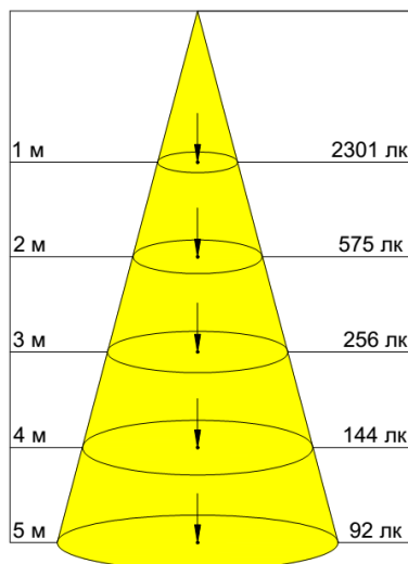
Микропризма 90°
