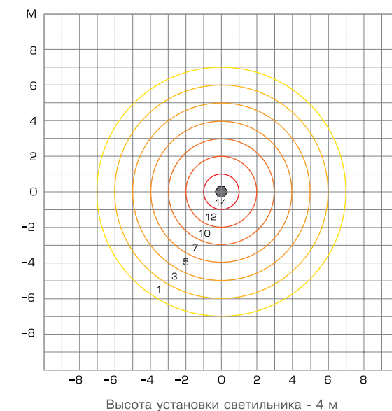
Диаграмма освещенности для светильника «Петродворец» 100 Вт с прозрачным стеклом, Ix
